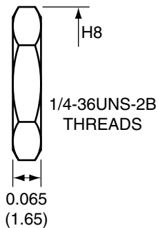
NUT
